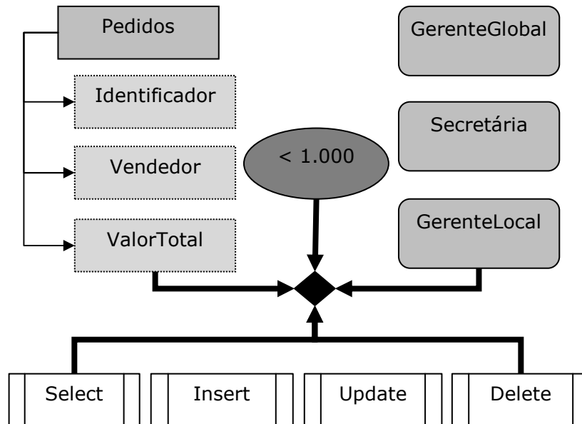
Figura 1 - Estrutura de uma Regra de Autorização
