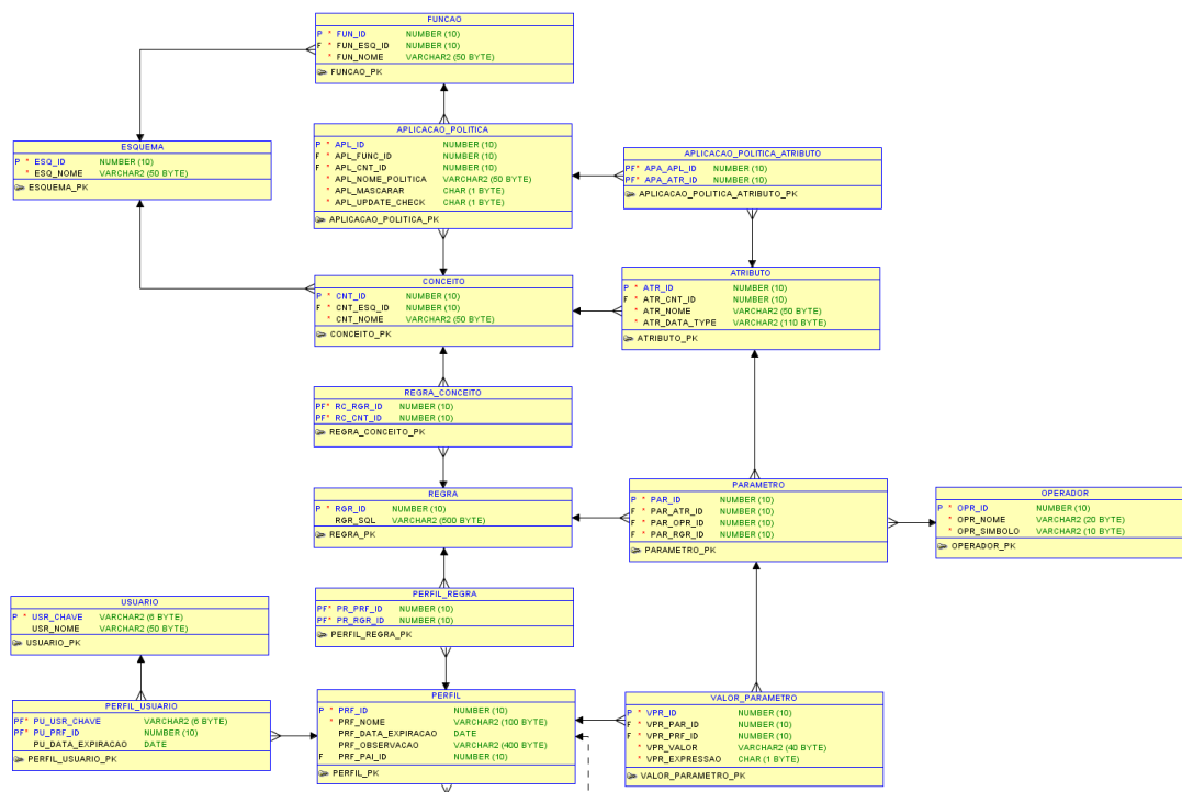
Figura 7 - Modelo relacional da implementação do framework
