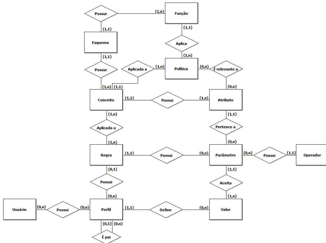
Figura 3 - Modelo de entidade e relacionamento do framework
